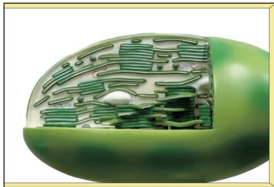
葉緑体の模式図
